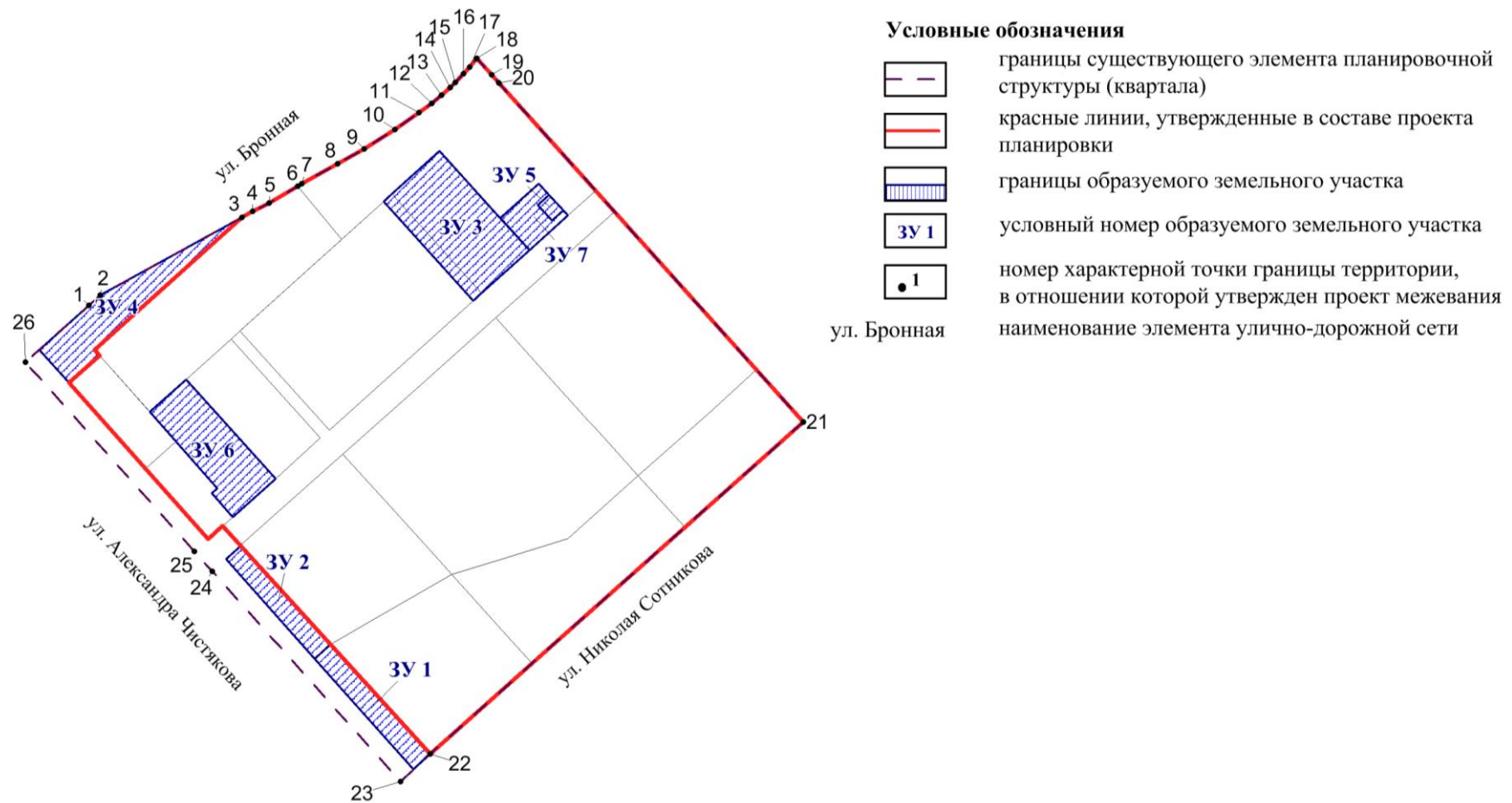
Чертеж межевания территории
